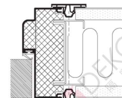
Solid Door and Doorframe
